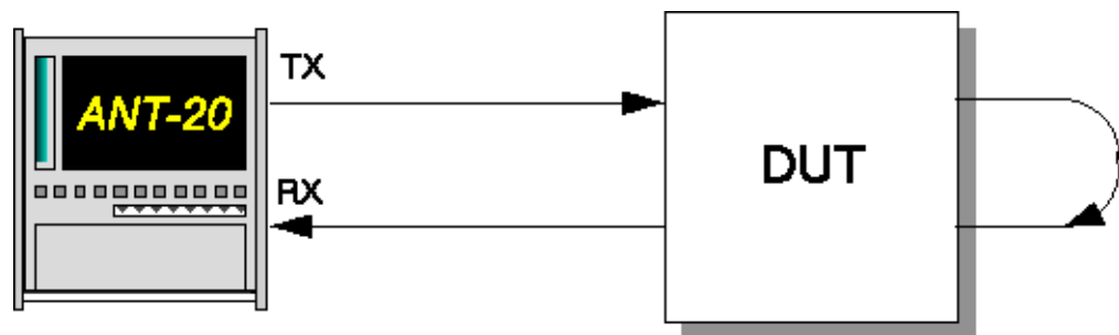
Bild A-1 Meßaufbau für MTJ-Messungen
