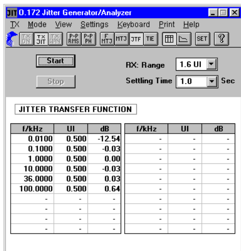
Bild A-13 JTF-Messungen: Tabellarische Ergebnisdarstellung
